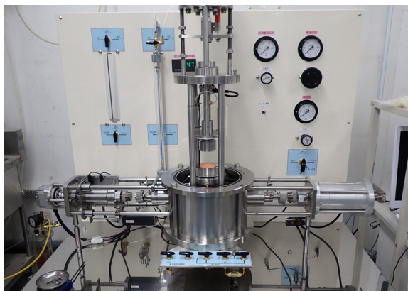
DSS: 繰返し単純せん断試験
