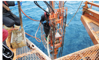
傾動自在用ボーリングマシン
