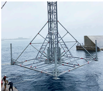
不陸調整装置「オクトパス」 (特許第7096561号)
