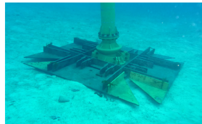
フレキシブル底盤【特許申請中】
