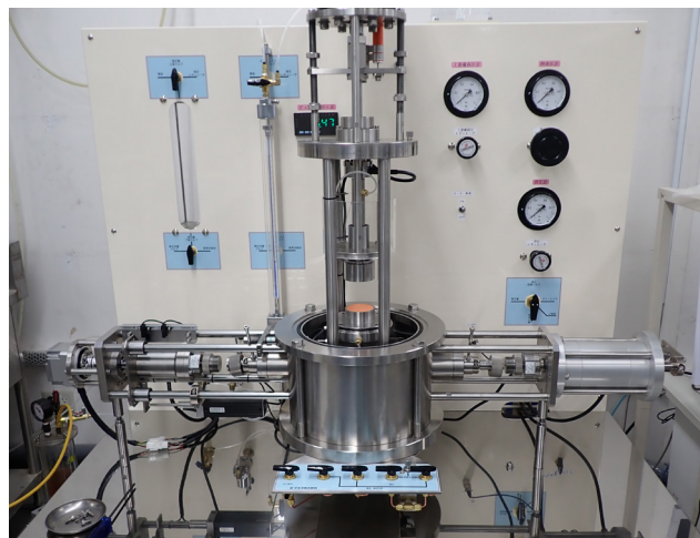
DSS: 繰返し単純せん断試験
