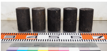
DSS: 繰返し単純せん断試験
