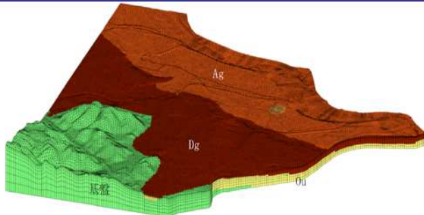
三次元有限要素モデル
