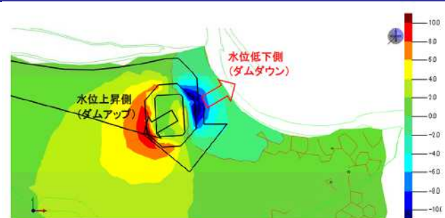
建設工事に伴う地下水位の変化
