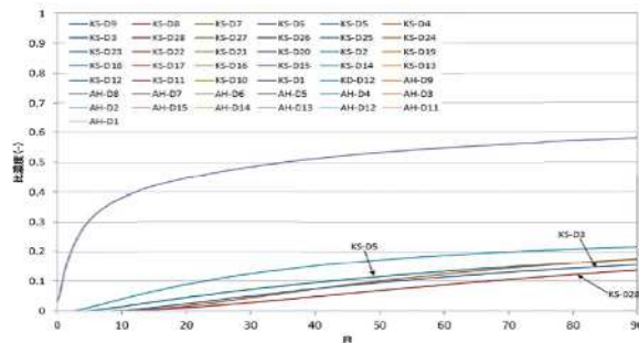
水源井戸における濃度の経時変化
