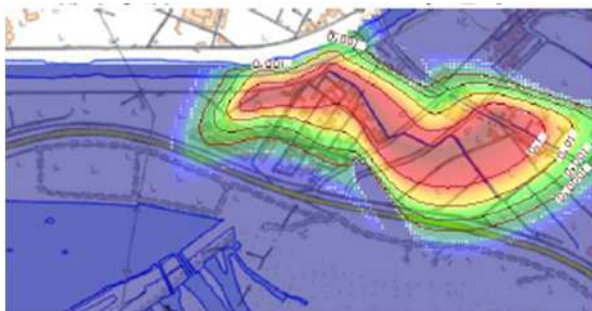
建設工事に伴う濁水の拡散状況の予測
